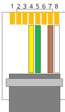
Рис. 3 — Схема распиновки
